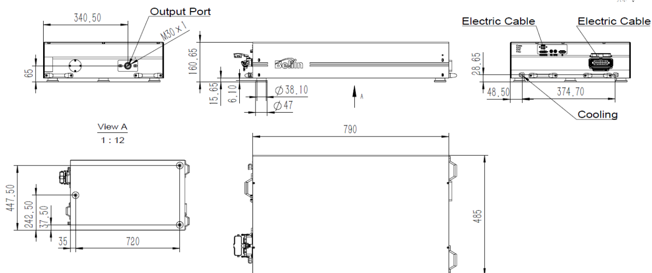
Amber NX UV-30 激光头外型尺寸图
