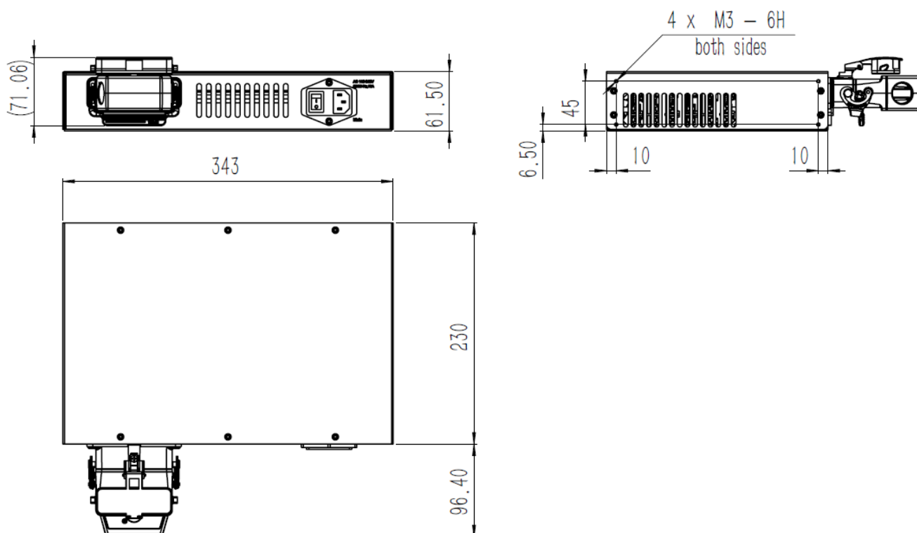
Amber NX UV-30 电源外型尺寸图
